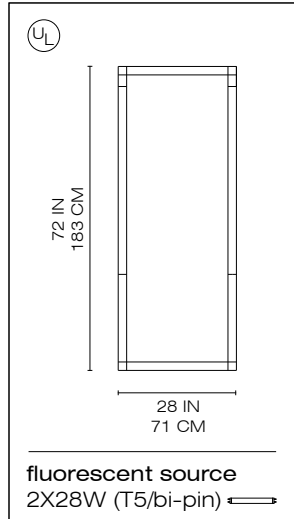
ADA floor 72
